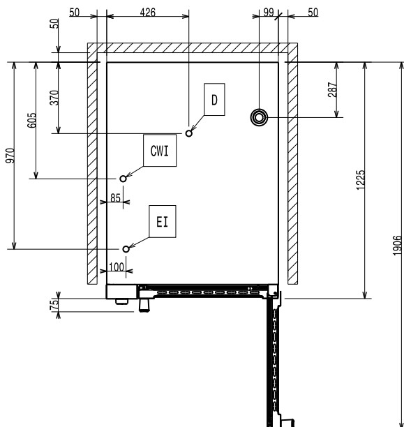
Boven aanzicht
